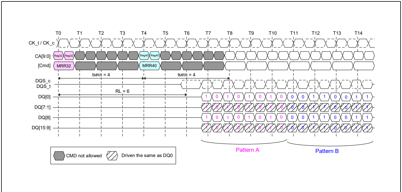
Figure 36 - DQ Calibration Timing
